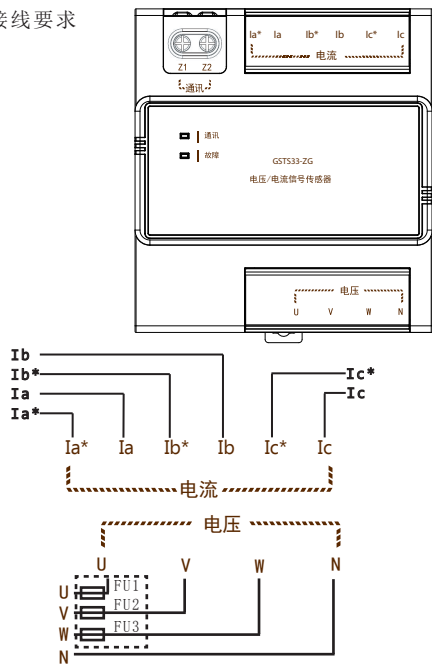
图一 电压电流测量接线方式
